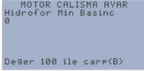
Şekil 3.6 Acil durum senaryosu aktif etme ekranı
