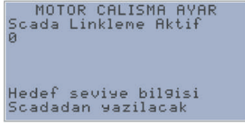
Şekil 3.8 SCADA Linkleme seçim ekranı
